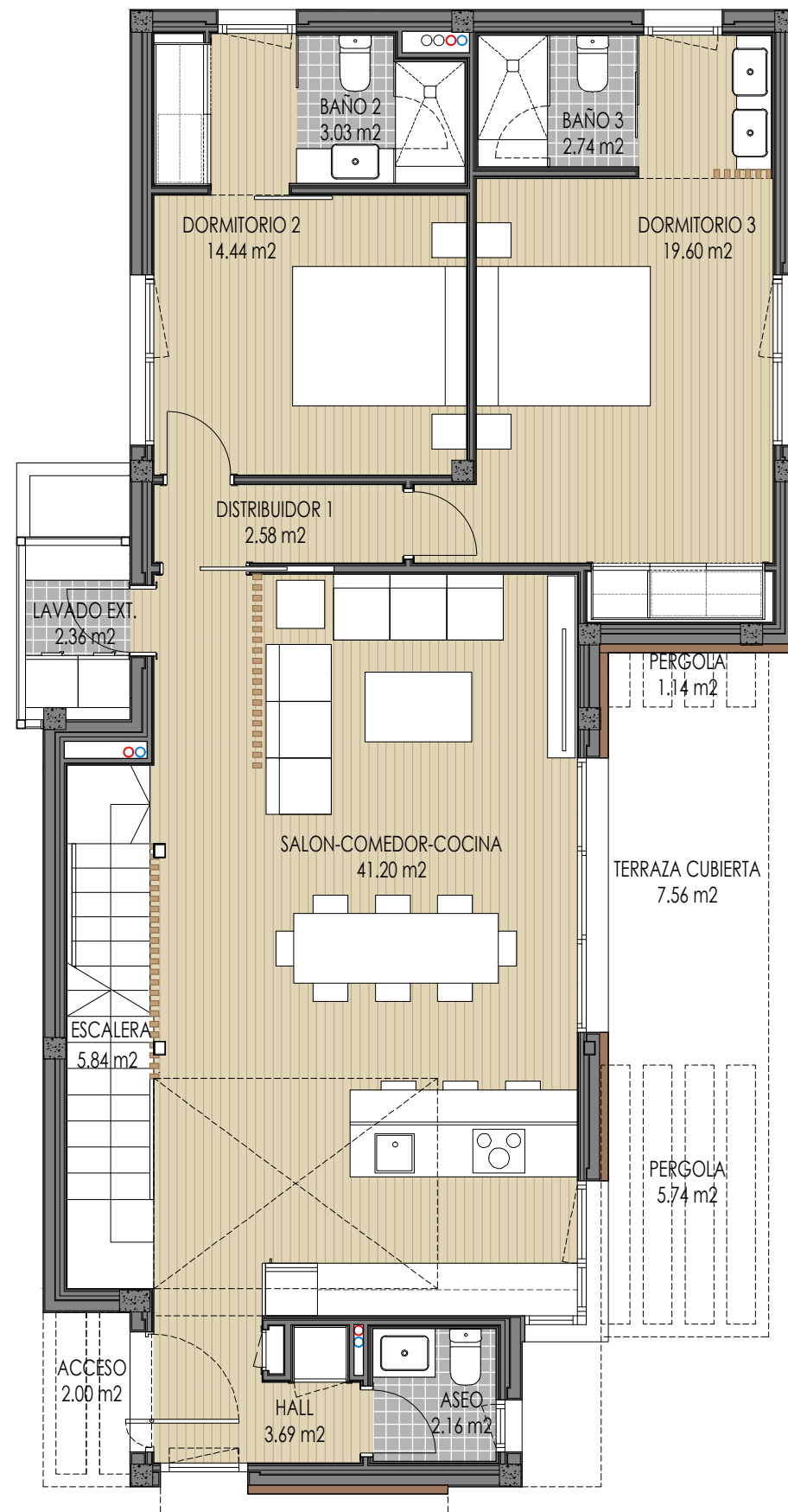
PLANTA BAJA
